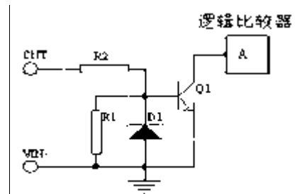
负逻辑控制电源内部原理图
