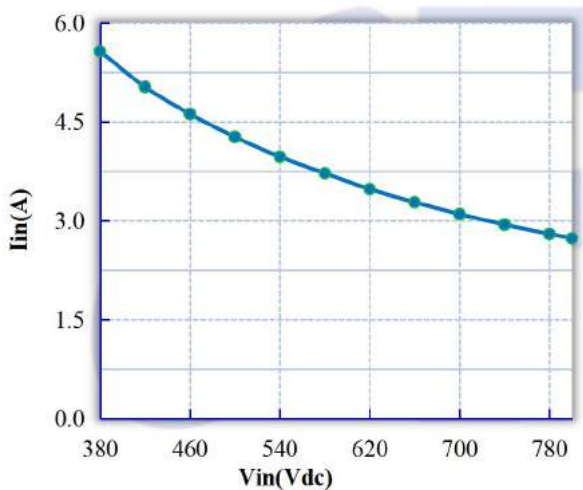
图(3):输入特性曲线
