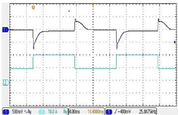
图(9):输出负载阶跃响应波形 (CH1:Vout,CH2:Iout;25%~50%~25%Load,2.5A/μs,输出端外接 1800μF 低 ESR 电解电容)
