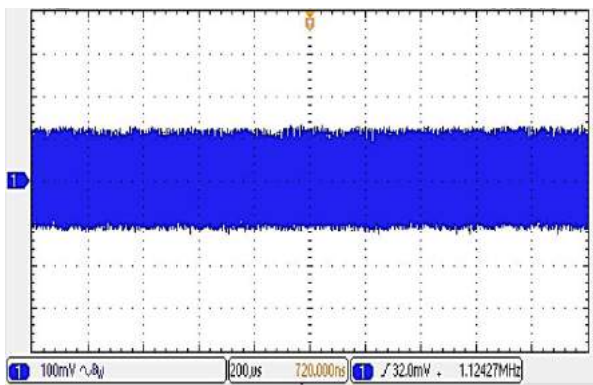
图(11):输出满载时的输出电压纹波 (200μs/div,输出端外接 1800μF 低 ESR 电解电容)
