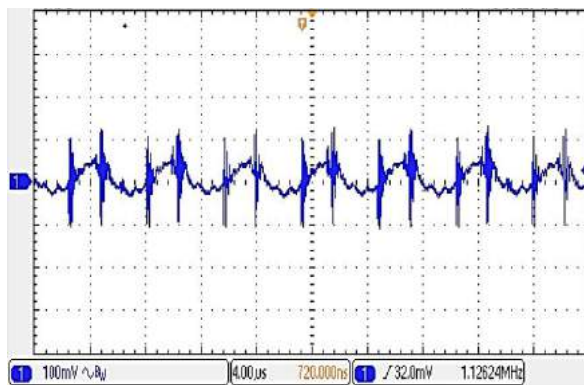
图(12):输出满载时的输出电压纹波 (4μs/div 输出端外接 1800μF 低 ESR 电解电容)
