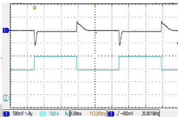
图(10):输出负载阶跃响应波形 (CH1:Vout,CH2:Iout;50%~75%~50%Load,2.5A/μs,输出端外接 1800μF 低 ESR 电解电容)
